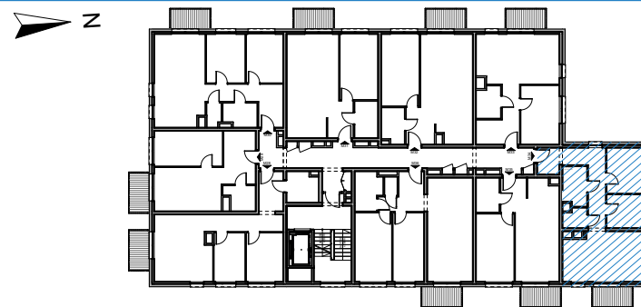
RZUT KONDYGNACJI
