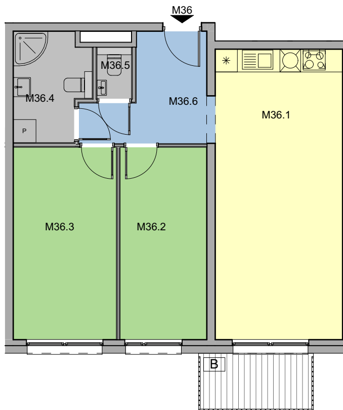
RZUT KONDYGNACJI
