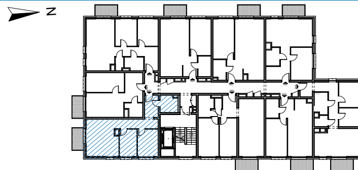
RZUT KONDYGNACJI
