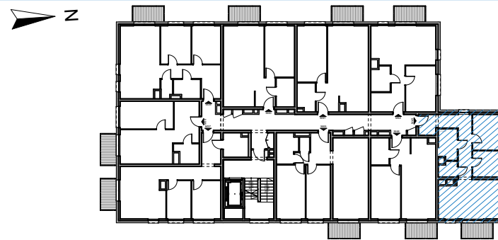
RZUT KONDYGNACJI
