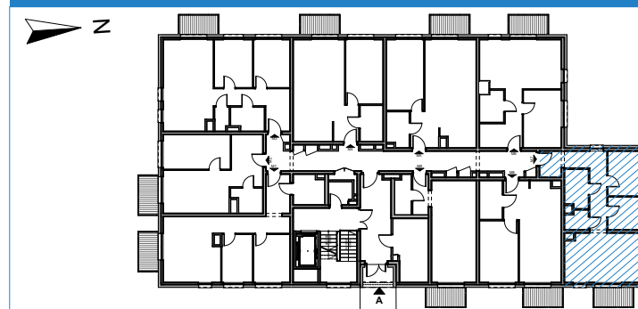
RZUT KONDYGNACJI
