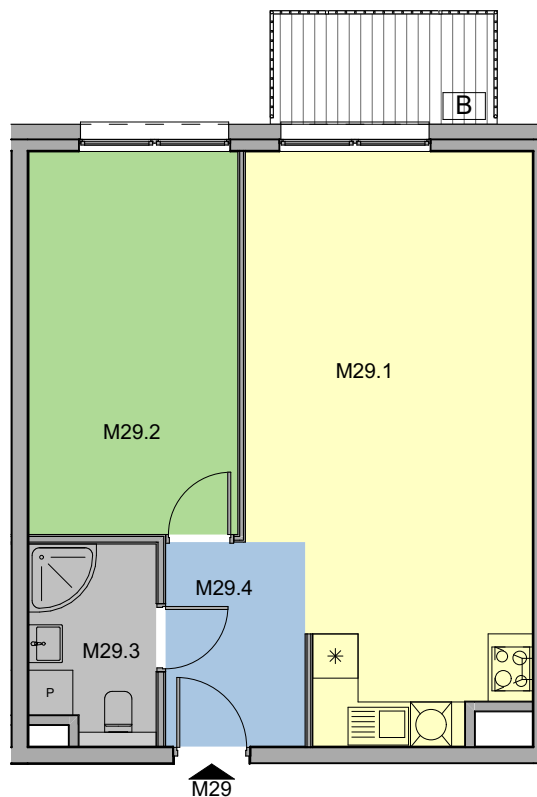
RZUT KONDYGNACJI
