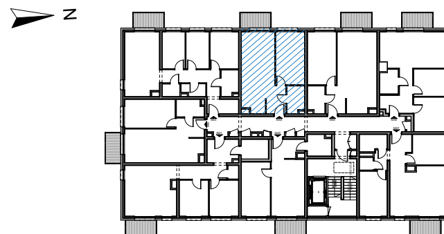
RZUT KONDYGNACJI
