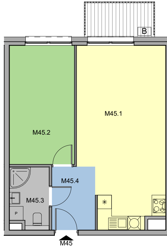
RZUT KONDYGNACJI
