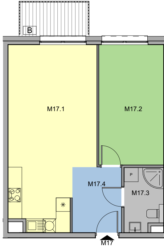
RZUT KONDYGNACJI
