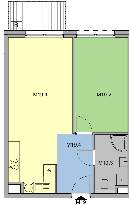
RZUT KONDYGNACJI
