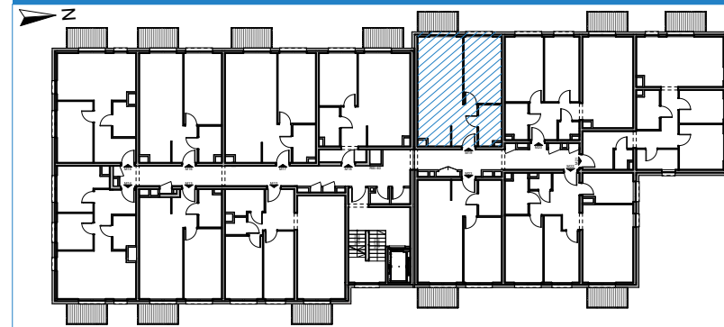
RZUT KONDYGNACJI
