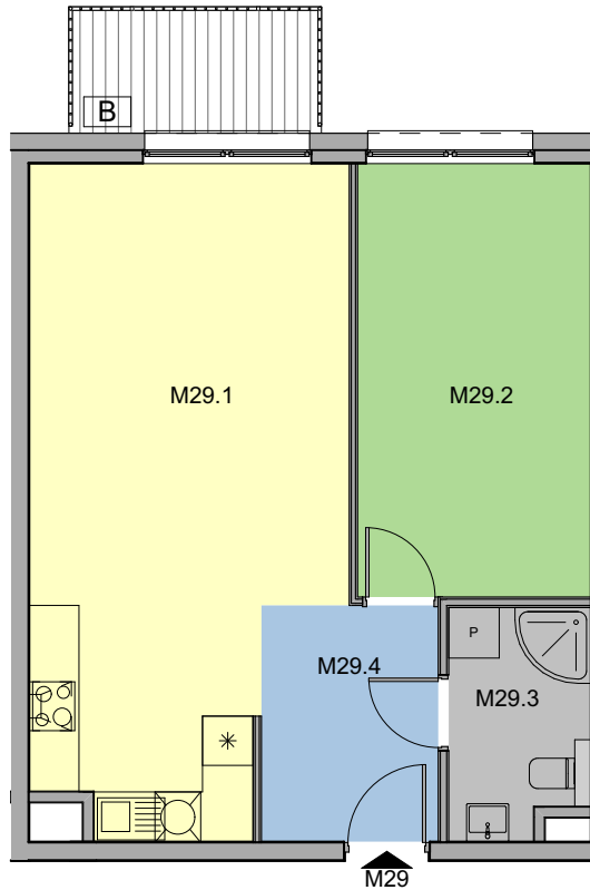
RZUT KONDYGNACJI
