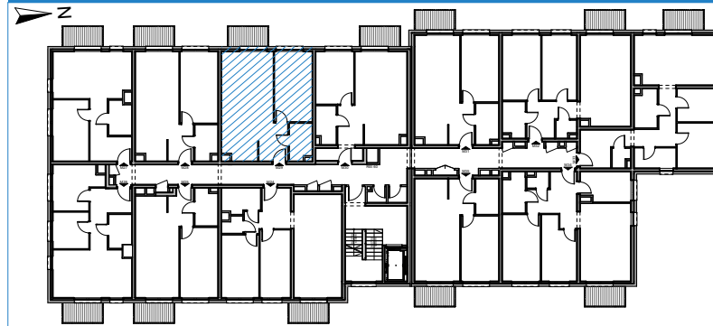
RZUT KONDYGNACJI
