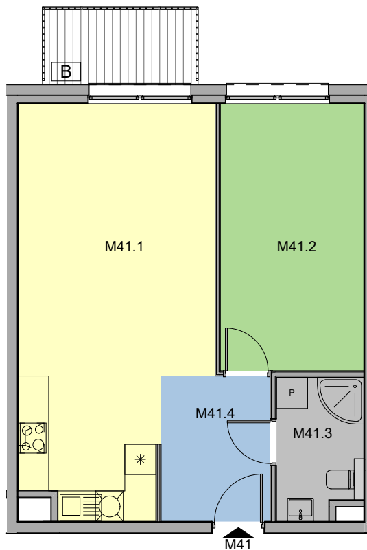
RZUT KONDYGNACJI
