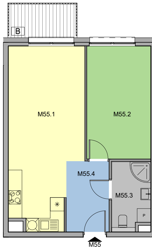
RZUT KONDYGNACJI
