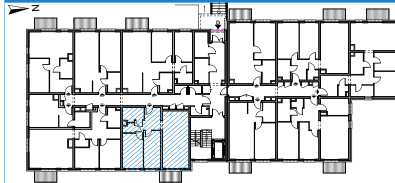
RZUT KONDYGNACJI
