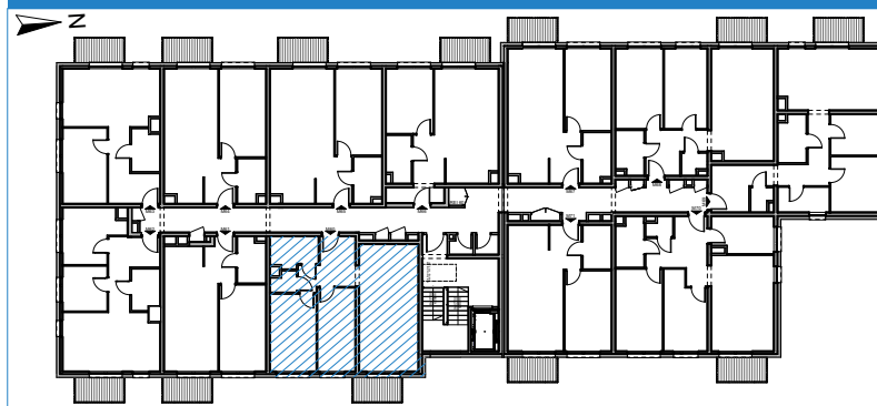
RZUT KONDYGNACJI
