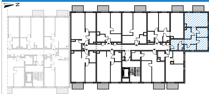
RZUT KONDYGNACJI
