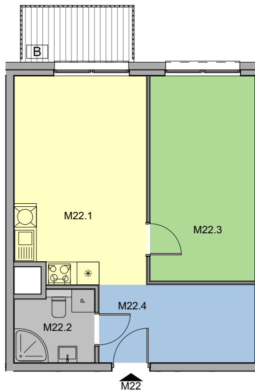
RZUT KONDYGNACJI
