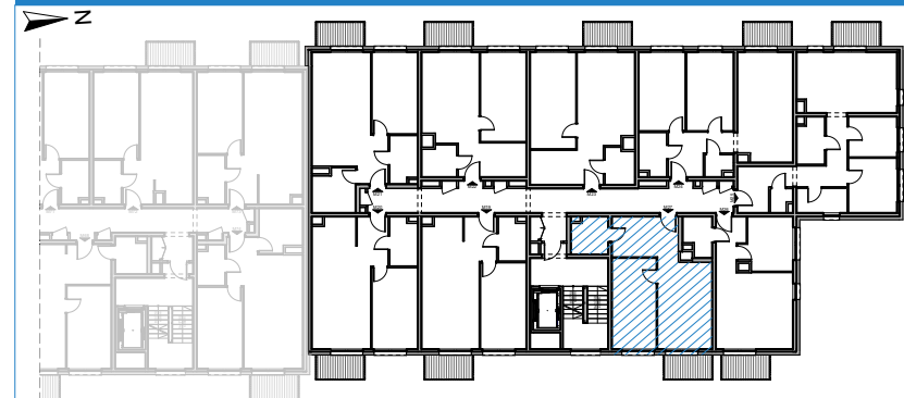
RZUT KONDYGNACJI
