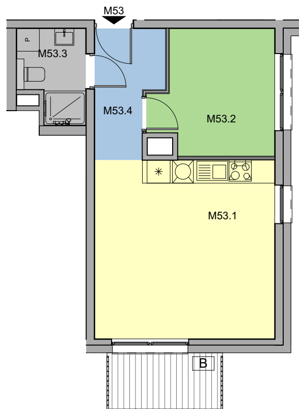
RZUT KONDYGNACJI
