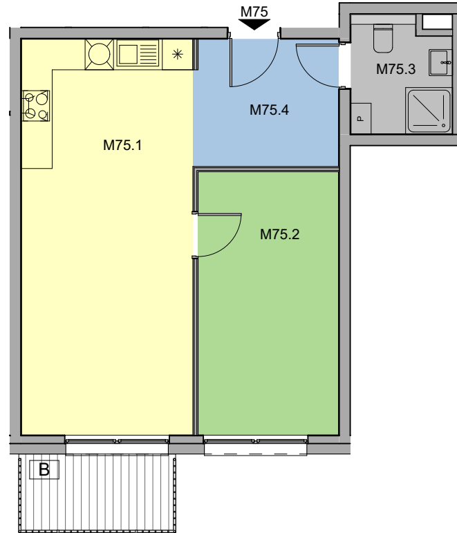
RZUT KONDYGNACJI
